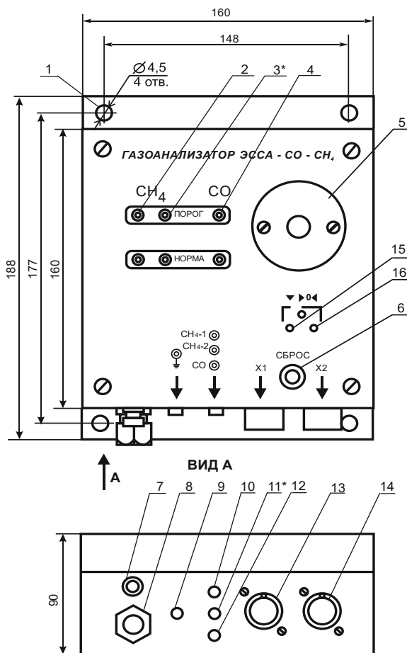
РИС. 2. БИС газоанализаторов ЭССА—СО-CH 4 /(2), габаритные и установочные размеры 1 – монтажное отверстие; 2 – светодиоды 1-го измерительного канала CH 4 ; 3* - светодиоды 2-го измерительного канала CH 4 ; 4 – светодиоды измерительного канала СО; 5 – детектор СО; 6 – кнопка СБРОС; 7 – предохранитель; 8 – кабельный ввод сетевого кабеля; 9 – гнездо «общий»; 10 – гнездо контрольной точки 1-го измерительного канала CH 4 ; 11* – гнездо контрольной точки 2-го измерительного канала CH 4 ; 12 – гнездо контрольной точки измерительного канала СО; 13 – разъем для подключения ИП CH 4 ; 14 – разъем для подключения внешних исполнительных устройств; 15 – резистор установки чувствительности измерительного канала СО; 16 - резистор установки нуля измерительного канала СО.
